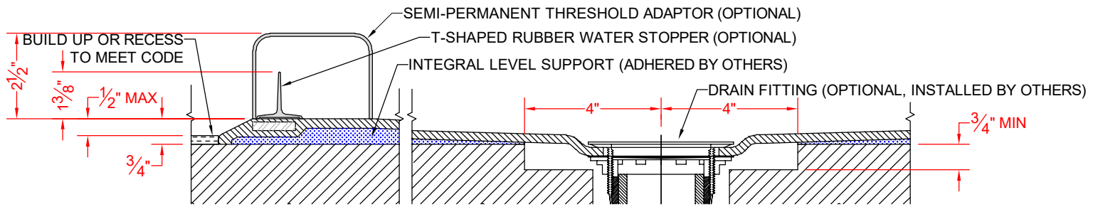
SECTION A-A - SCALE: 3" = 1'-0"
