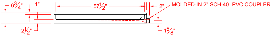
FRONT ELEVATION - SCALE: \frac{3}{8}'' = 1'-0''
