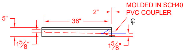
FRONT ELEVATION - SCALE: \frac{3}{8}'' = 1'-0''
