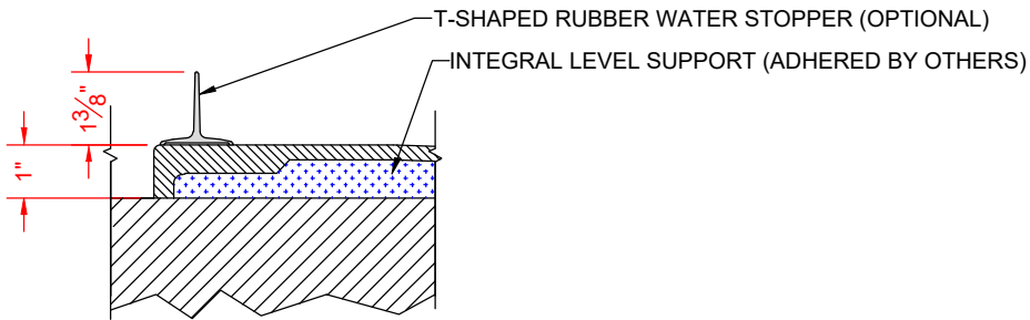
SECTION B-B - SCALE: 3" = 1'-0"
