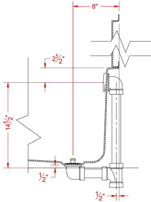
SECTION A-A - SCALE N.T.S. TUB DRAIN/OVERFLOW DETAIL
